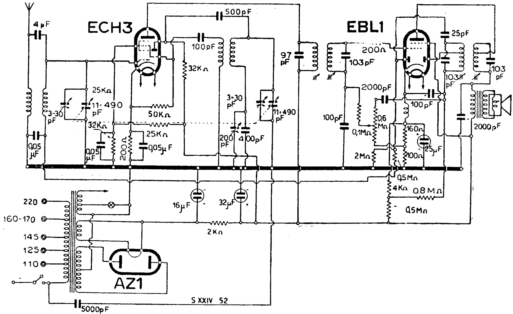
PHILIPS RADIO - MOD. « ROMA »
